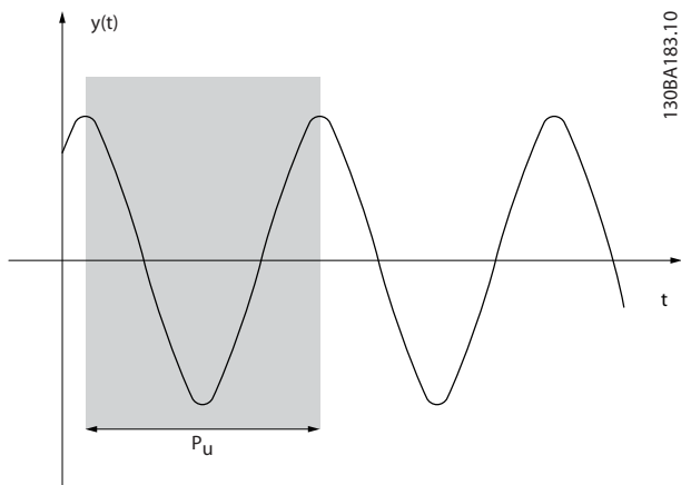
Рисунок 2.26 Система на границе устойчивости
