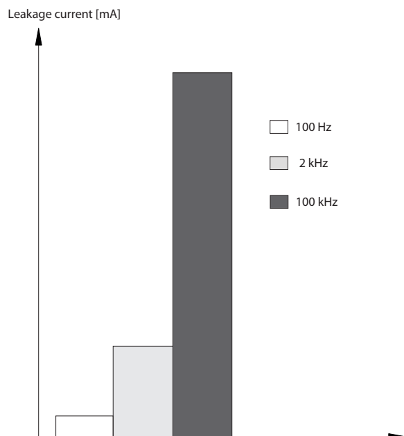
Рисунок 2.32 Влияние частоты отключения датчика остаточного тока (RCD) на величины реагирования/измеряемые величины
